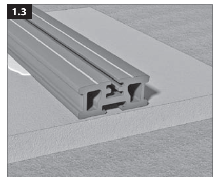
1.3 Montage auf Betonplatten/liegenden Randsteinen (min. 40 x 40 x 4 mm)
