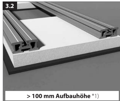
3.2 Montage auf Betonplatten. (min. 40 x 40 x 4 mm)
